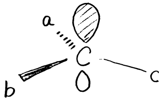
sp^2 と sp^3 の間
