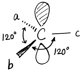
sp^2 混成
