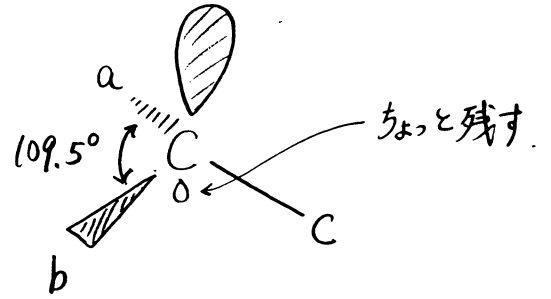
sp^3 混成
