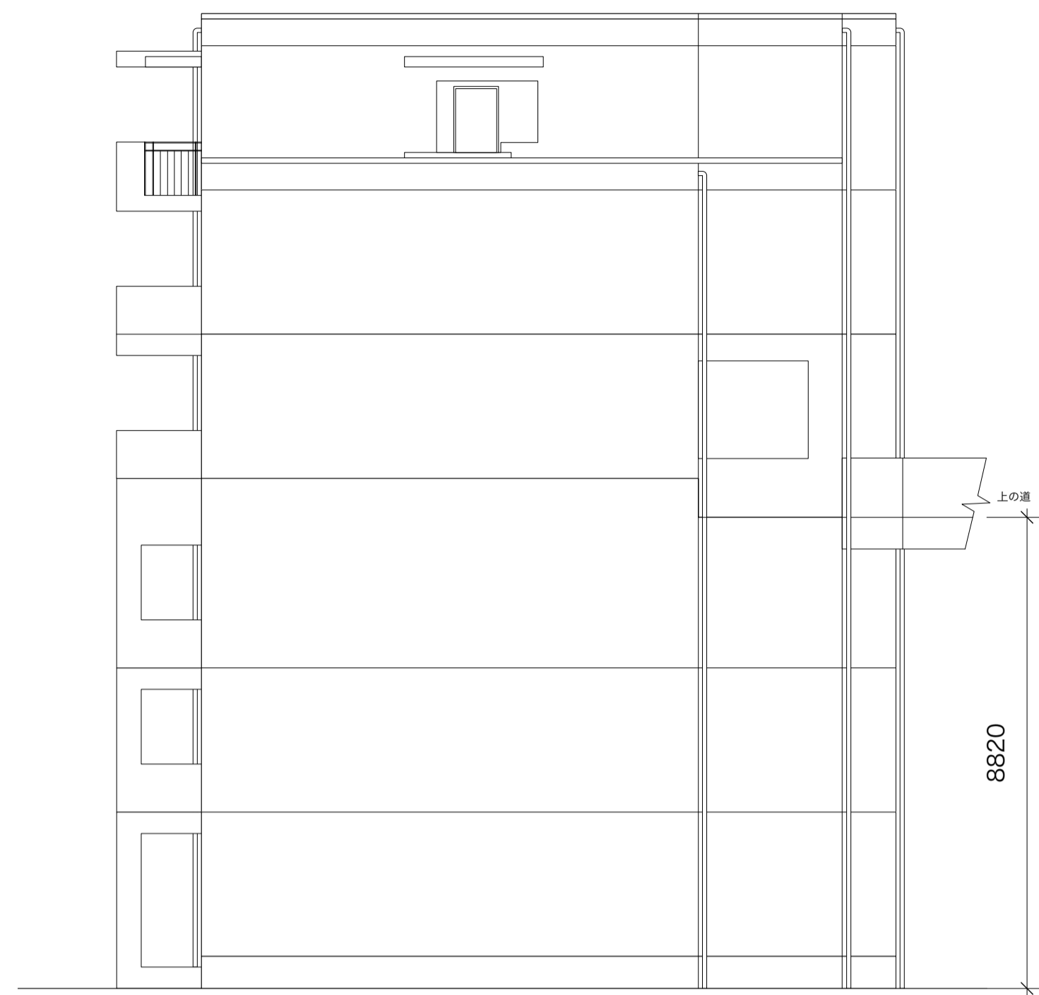
北側立面図
